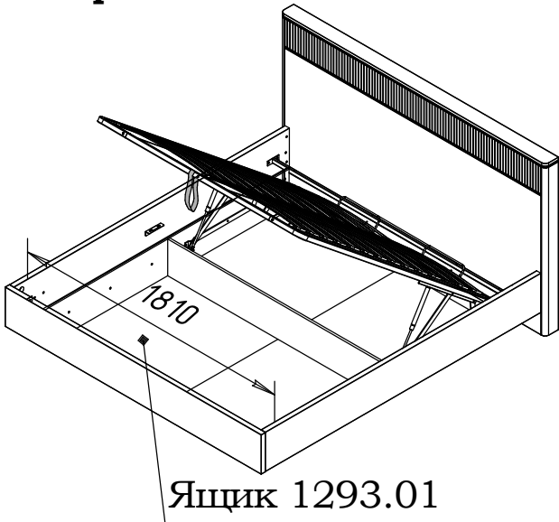
Кровать 83.202.00.00-01
