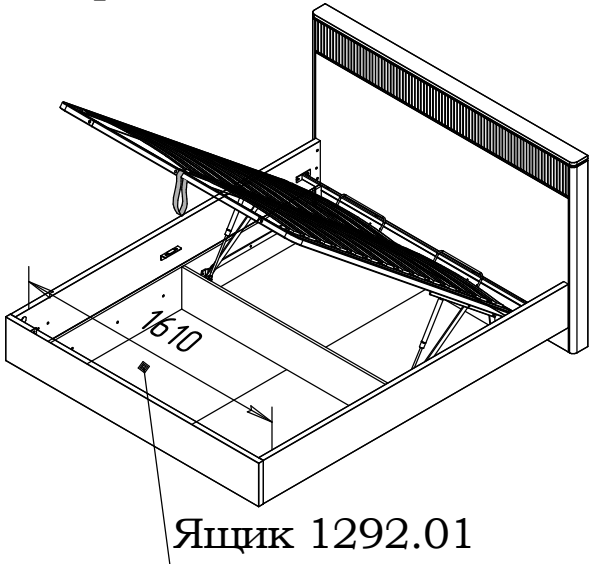
Кровать 83.201.00.00-01
